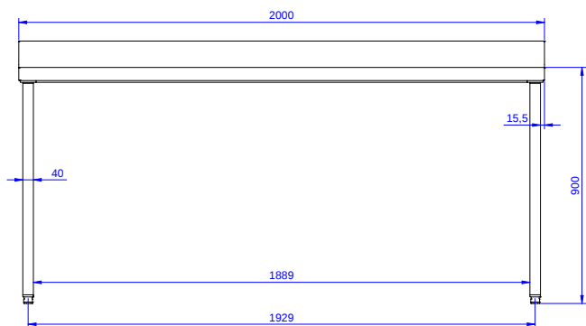
Bočna/o
